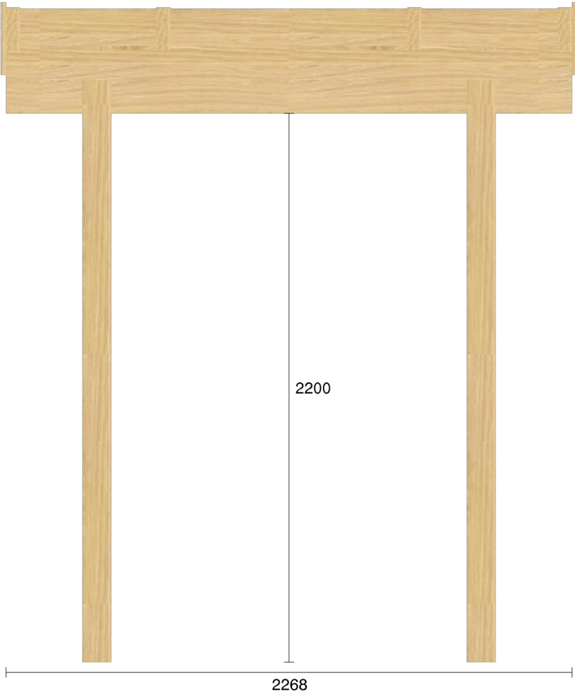
Elevationsvy front yttermått
